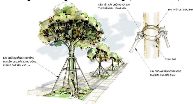
Hình 18. Phòng và giảm thiểu thiệt hại cho cây xanh bằng thanh chống thép
