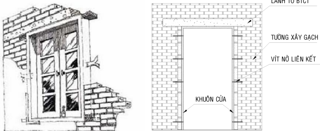
Hình 14. Gia cố khuôn cửa
