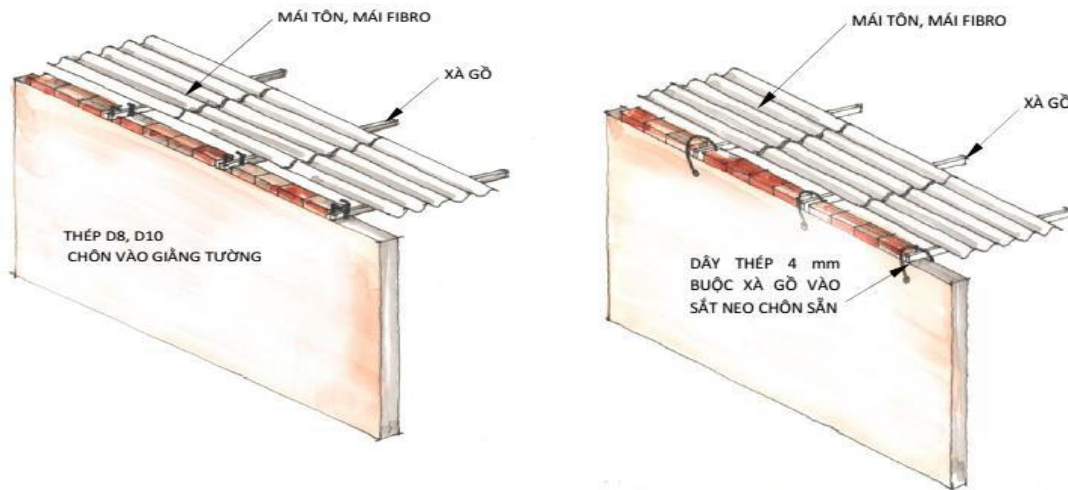
Hình 13. Neo buộc xà gỗ mái tôn
